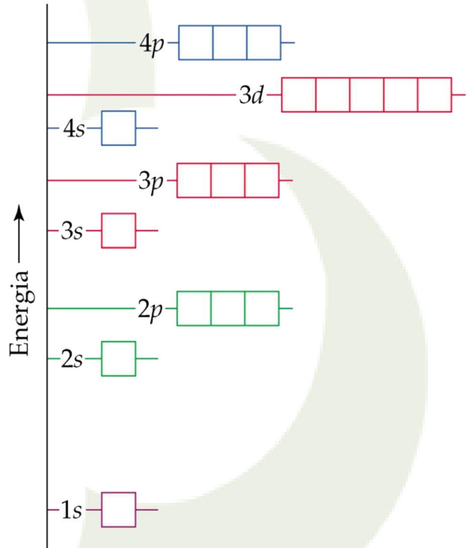
Átomos Polieletrônicos
